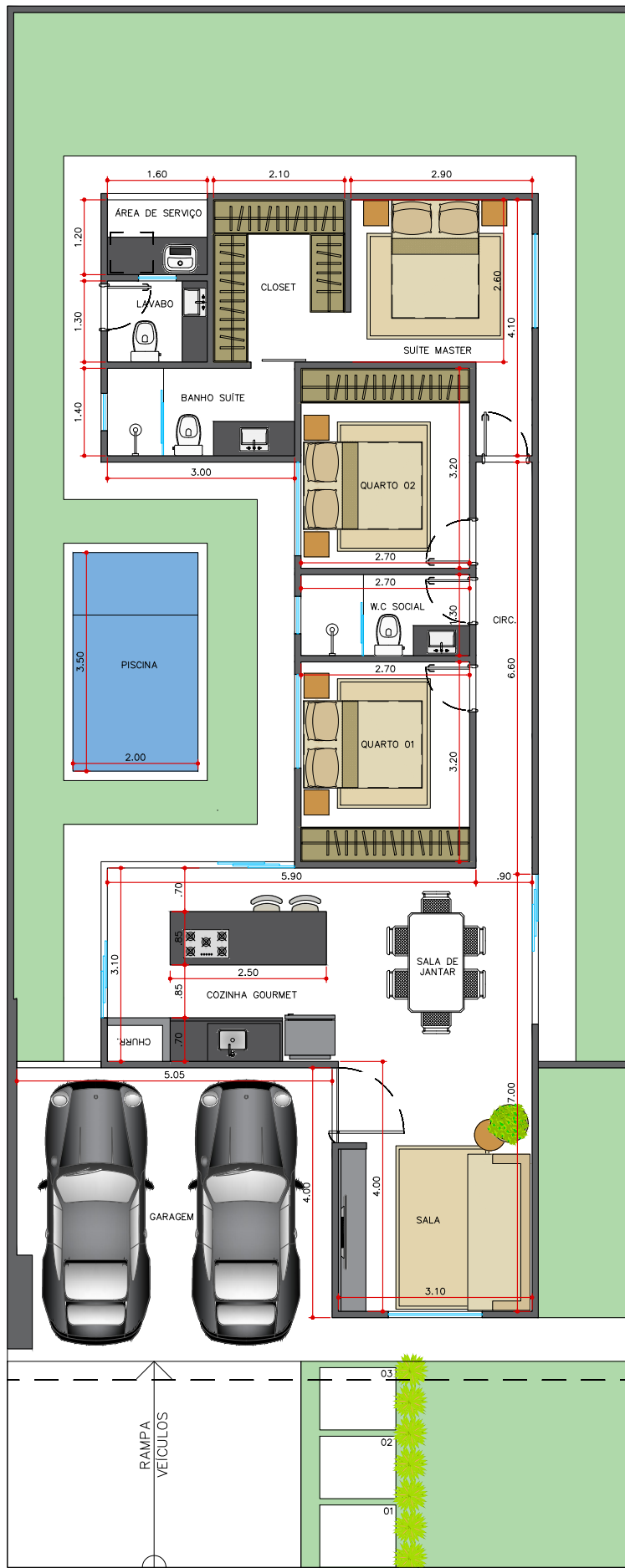
LAYOUT - 112,30 m 2 ESCALA sem escala
